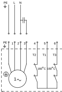
Рис. 3 Монтажная электросхема для насосов с однофазными электродвигателями
