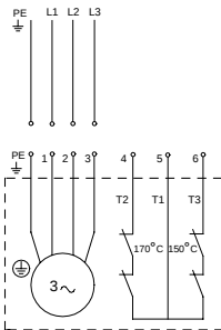
Рис. 4 Монтажная электросхема для насосов с трехфазными электродвигателями
