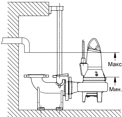
Рис. 5 Уровни пуск и останов
