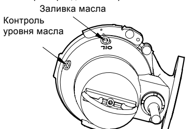
Рис. 10 Отверстия для заправки насоса смазкой
