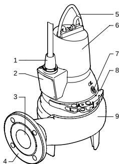
Рис. 1 Насос SE1.50.65
