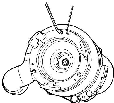
Рис. 9 Вид насоса со стороны всасывания
