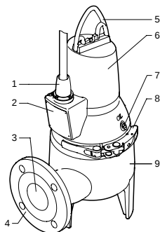
Рис. 2 Насос SEV.65.65
