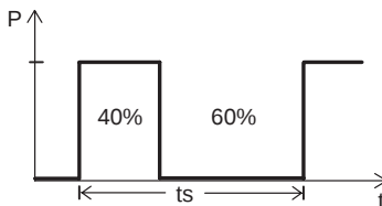
Рис. 6 Режим работы S3
